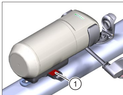
Fig. 5: Sistema FIDLOCK® sbloccato
