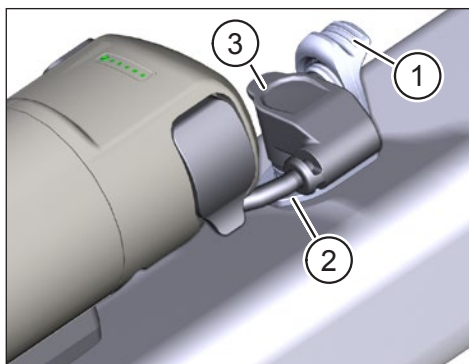
Abb. 8: Verbinden Sie das Verbindungskabel mit dem Ladeanschluss
